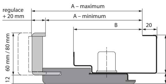
průřez zárubně PROJEKT Premium
