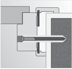
montáž na pěnu a kotvy do zdivné stěny
