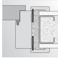
montáž na pěnu do stěny ze sádrokartonu
