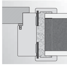
montáž na pěnu do zdivné stěny
