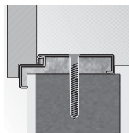
rohová zárubeň velká montáž pomocí šroubů
