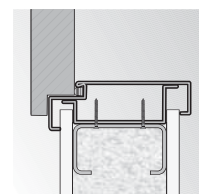
rohová zárubeň velká montáž na sádrokartonovou stěnu
