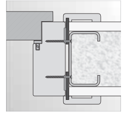
montáž na vrutky do stěny ze sádrokartonu
