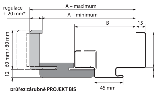
průřez zárubně PROJEKT BIS
